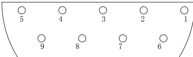
9针D型母头俯视图
